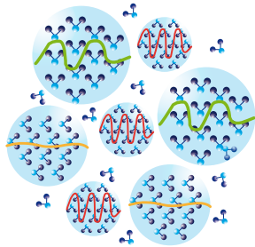
Coherence Domains
